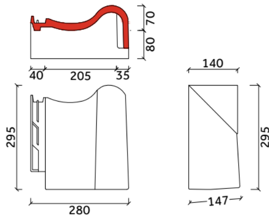
Chaperongevelpan rechts 90° De Nieuwe Hollander Plus
