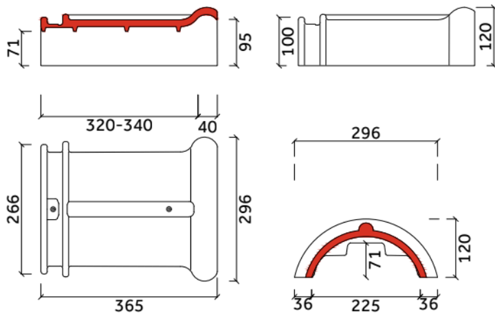
halfronde vorst Plus
