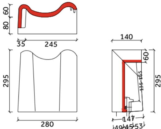
Chaperongevelpan links 90° De Nieuwe Hollander Plus
