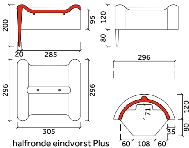
halfronde beginvorst Plus
