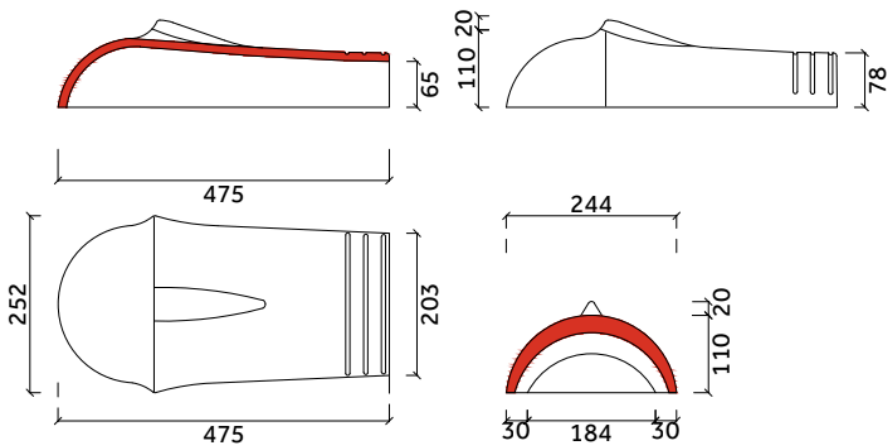
hoekkeperbegin schubvorst Plus
