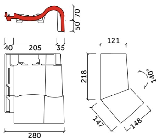
knikgevelpan rechts 140° De Nieuwe Hollander Plus
