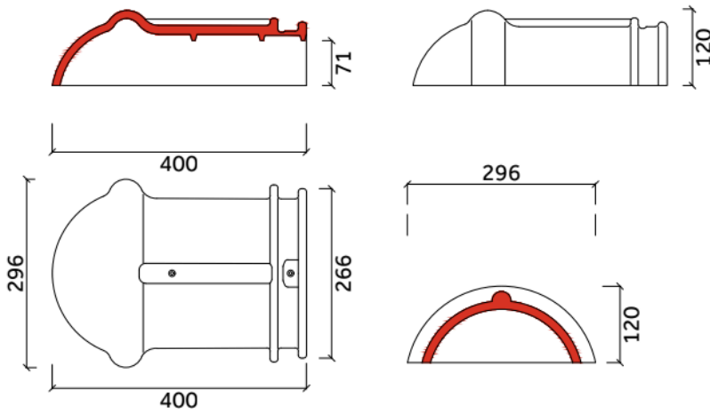
halfronde hoekkeperbeginvorst Plus
