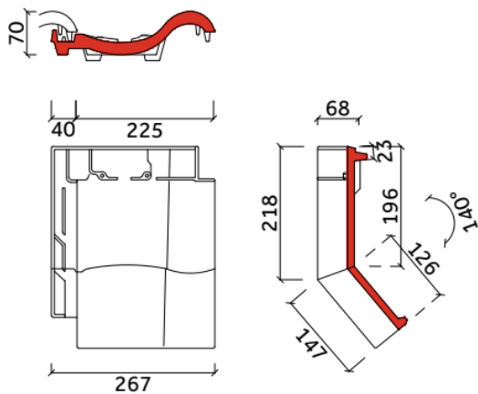
knikpan 140° De Nieuwe Hollander Plus
