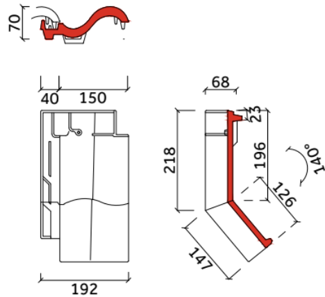
2/3 knikpan 140° De Nieuwe Hollander Plus
