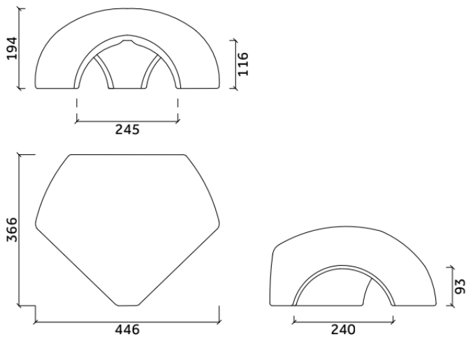
broekstuk 1x halfronde vorst Plus + 2x Schubvorst Plus
