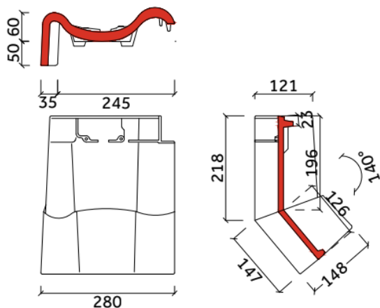
knikgevelpan links 140° De Nieuwe Hollander Plus
