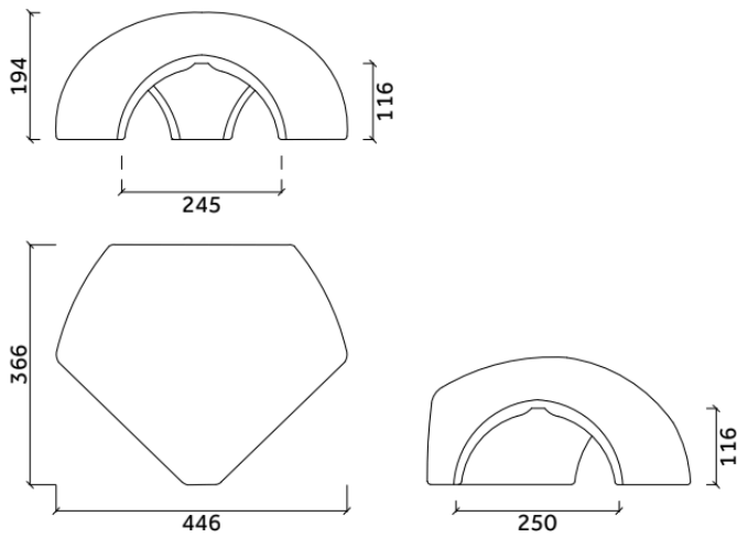
broekstuk 3x halfronde vorst Plus
