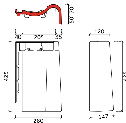
gevelpan rechts
