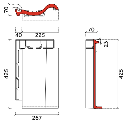
onderpan
