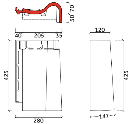
ondergevelpan rechts
