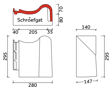
chaperongevelpan rechts 90°
