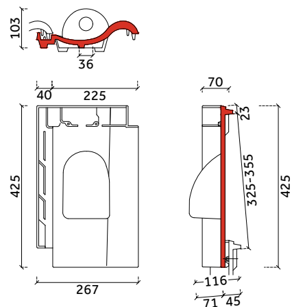
huismussenpan
