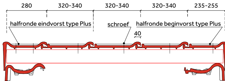
Nok verdeling halfronde vorst type Plus
