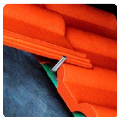
Euro-panhaak Frankfurter
