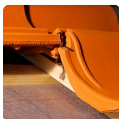
Euro-panhaak OVH 206
